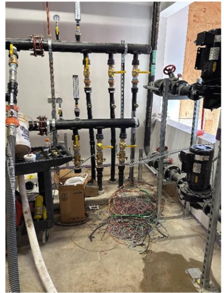
Geothermal Loop Glycol Fill
